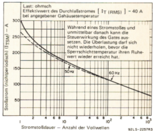
Bild 4: Stoßstrom in Abhängigkeit von der Stromstoßdauer
